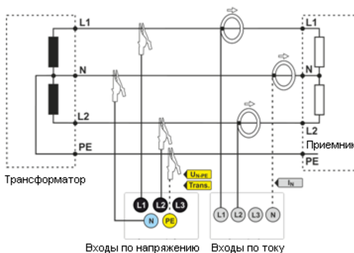
Рис. 17. Схема подключения – сеть с расщеплённой фазой (двухфазная).
