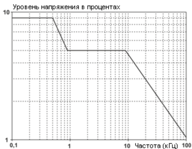
Рис. 47. Допустимые уровни управляющих сигналов.
